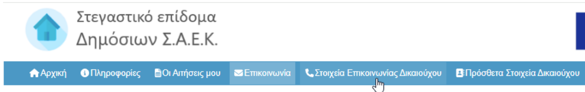
Εικόνα 80 Στοιχεία επικοινωνίας
