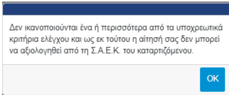
Εικόνα 78 Προειδοποιητικό Μήνυμα
