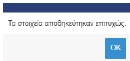
Εικόνα 85 Επιτυχής αποθήκευση
