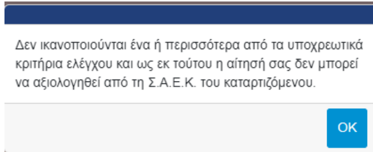
Εικόνα 47 Προειδοποιητικό Μήνυμα
